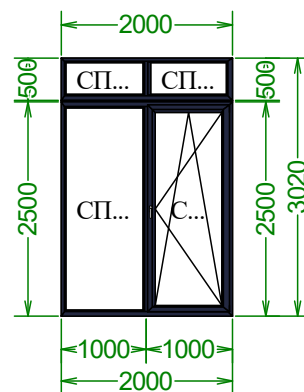
3020×2000 мм 1 шт
