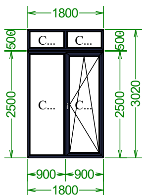
3020×1800 мм 3 шт
