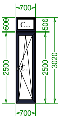
3020×700 мм 1 шт
