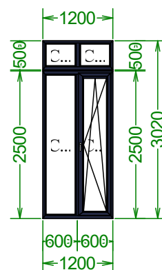
3020×1200 мм 1 шт
