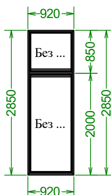
2850×920 мм 1 шт
