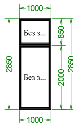
2850×1000 мм 1 шт
