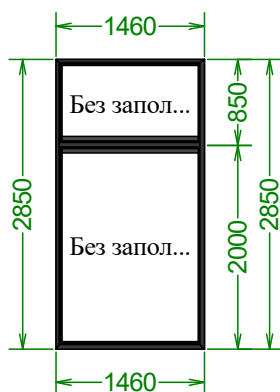
2850×1460 мм 1 шт
