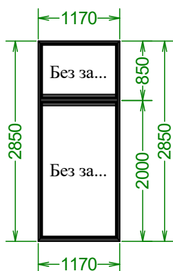
2850×1170 мм 1 шт
