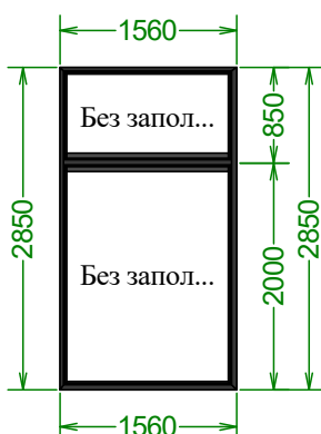
2850×1560 мм 4 шт
